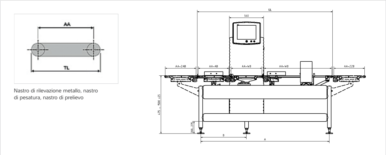
La figura mostra come esempio un sistema combinato con direzione di trasporto da sinistra verso destra.
